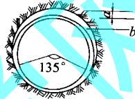
图 6.3.7 超挖示意图
